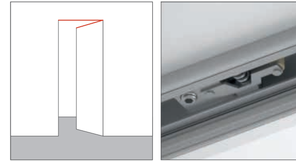
매립형 도어클로저(홀드/오픈장치)
